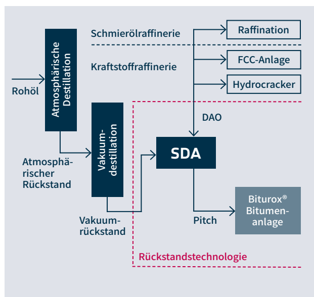
SDA-Anlage als Bestandteil einer modernen Rückstandstechnologie
